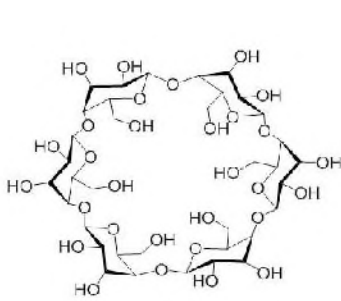
\alpha -Cyclodextrin
