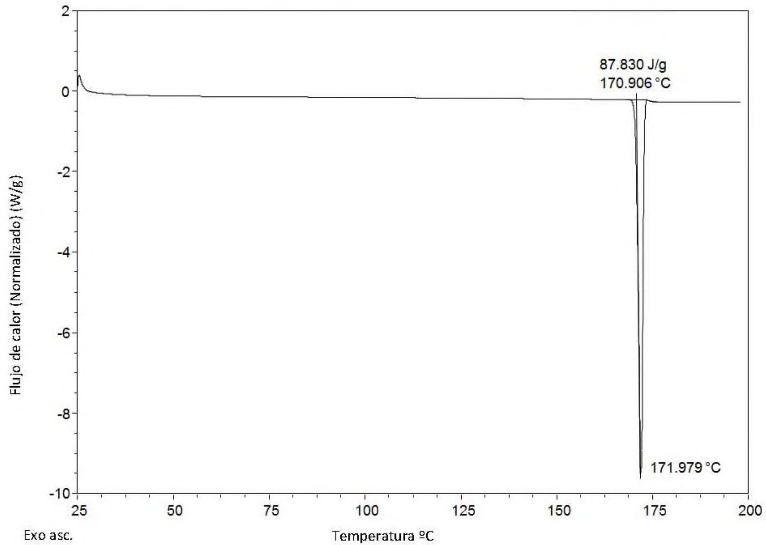
Figura 2: Termograma de DSC para la Forma A cristalina.
