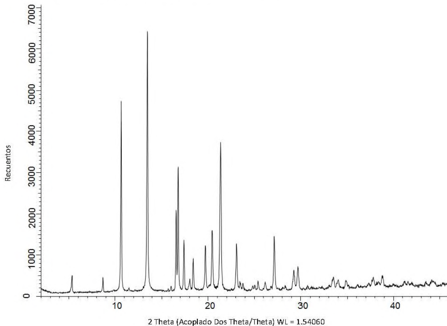
Figura 4: Patrón de difracción de rayos X en polvo para la Forma B cristalina.
