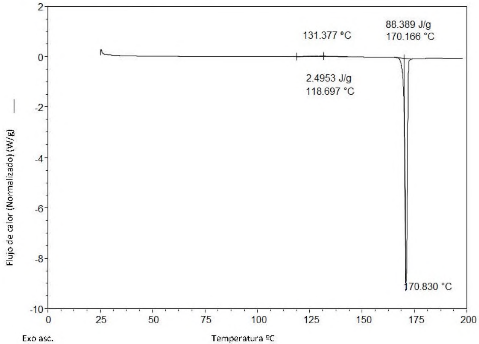
Figura 5: Termograma de DSC para la Forma B cristalina.
