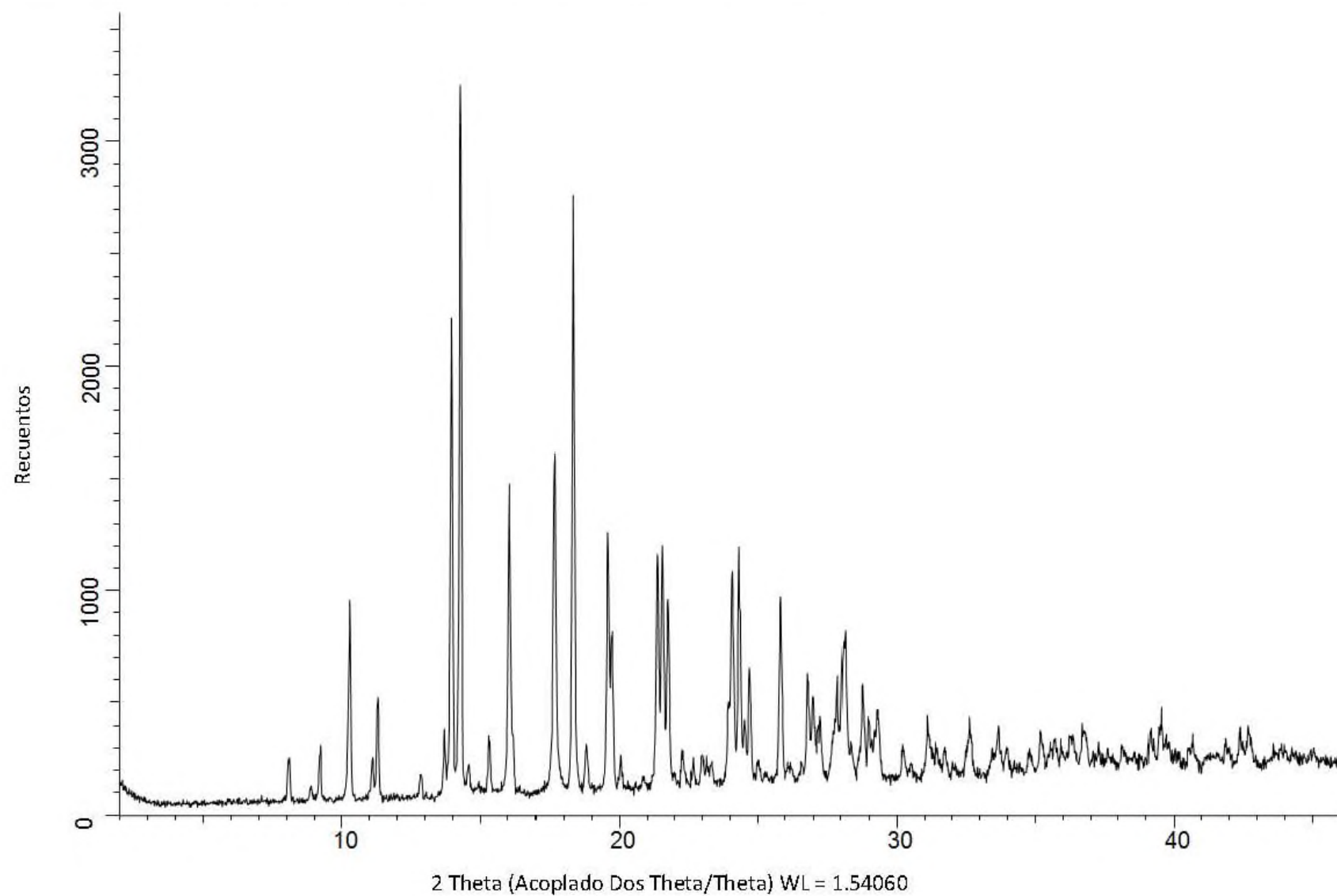
Figura 6: Patrón de difracción de rayos X en polvo para la Forma H A cristalina.
