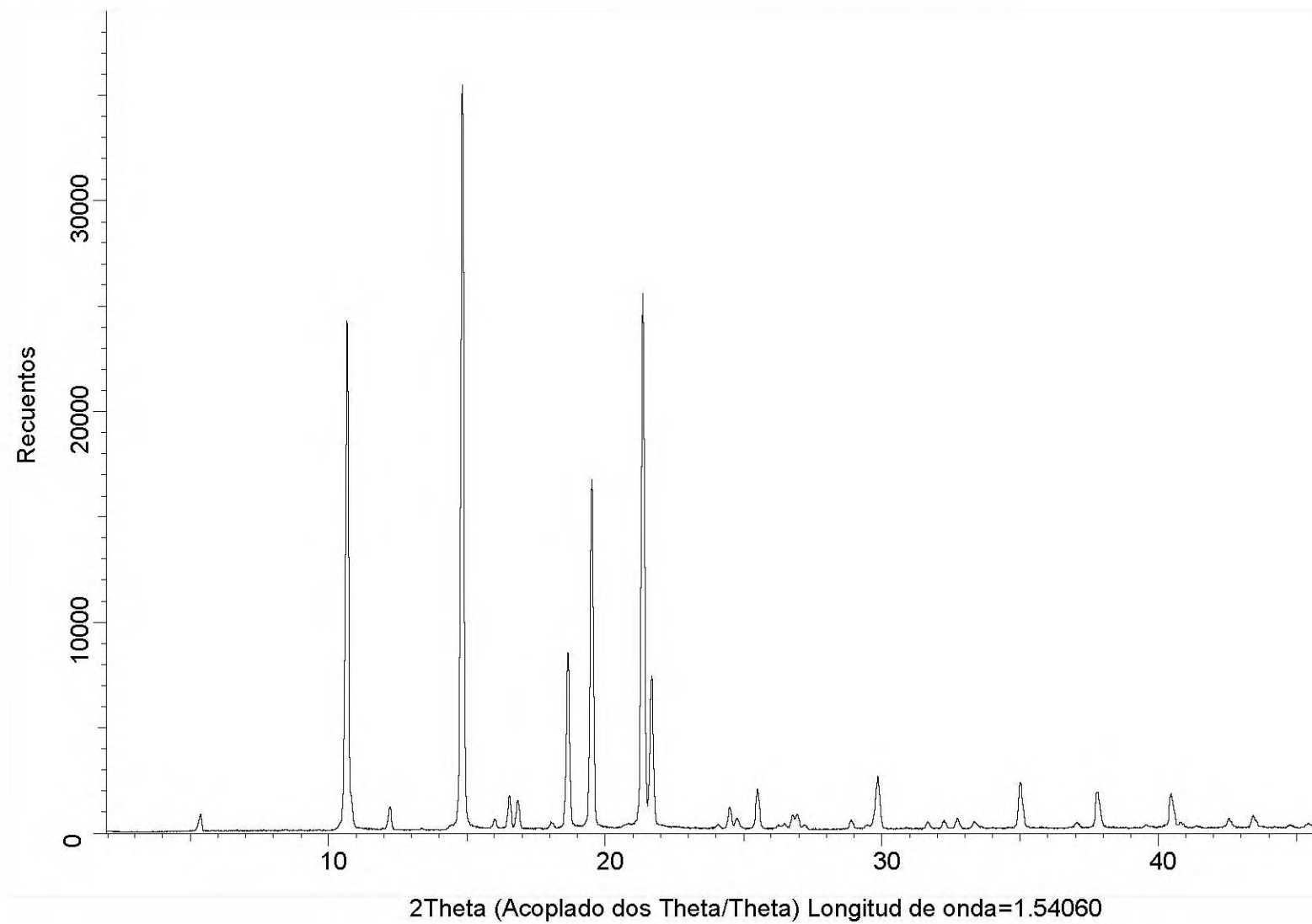
Figura 1: Patrón de difracción de rayos X de polvo del Compuesto 1 cristalino (Forma A)
