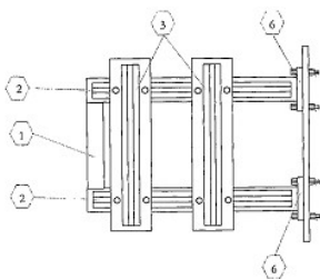
Figura No. 1 Vista superior de la mesa del motor eléctrico.
