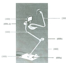
Figura 2. Partes de la ortesis activa.
