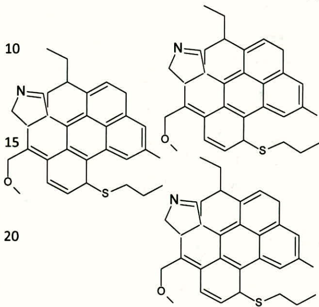
ASFALTENOS (a)
