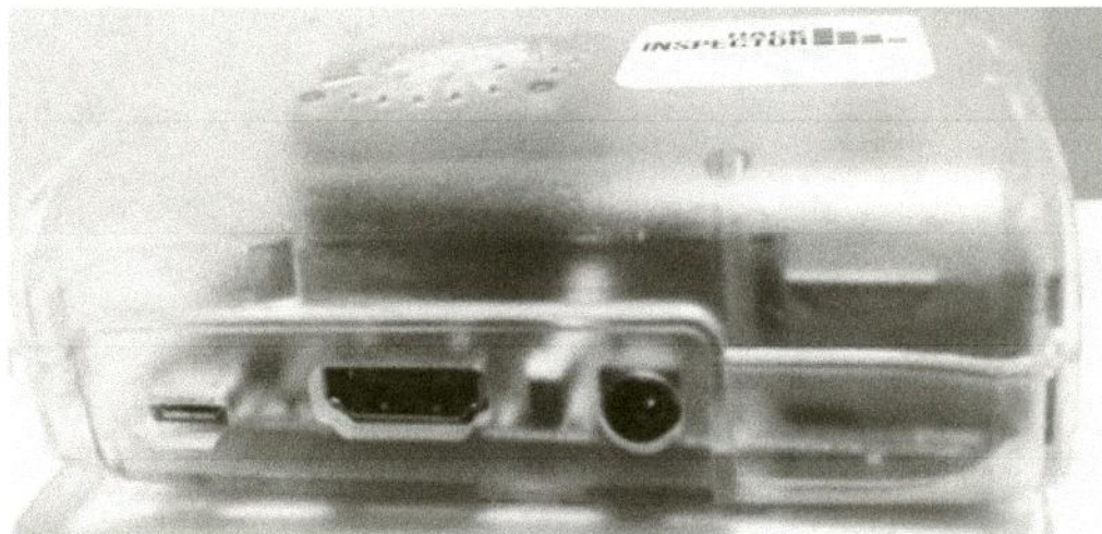
Imagen 24: Dispositivo lateral 2 (Se evidencia de izquierda a derecha puerto de alimentación, puerto HDM y, puerto de audio).
