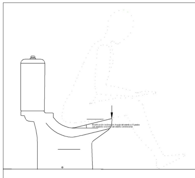
Grafica 2. ERGOVAC - Sanitario modificado según la propuesta
