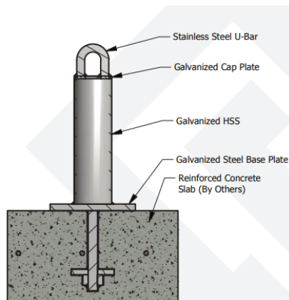
Ilustración 1: Sistema de protección contra caídas del documento D2.
