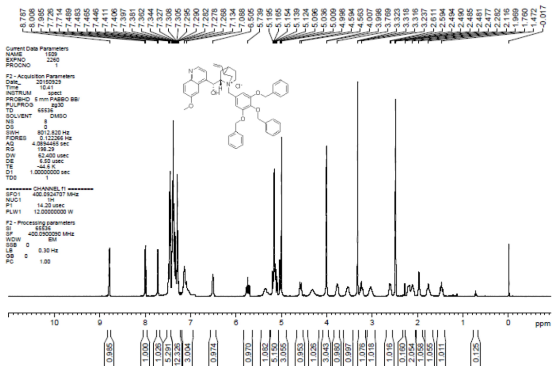
Figura 1: espectros de ^1\text{H} RMN de catalizador de transferencia de fase quiral (IIIa-13-1) preparado en el Ejemplo 1 en \text{DMSO-d}_6 .
