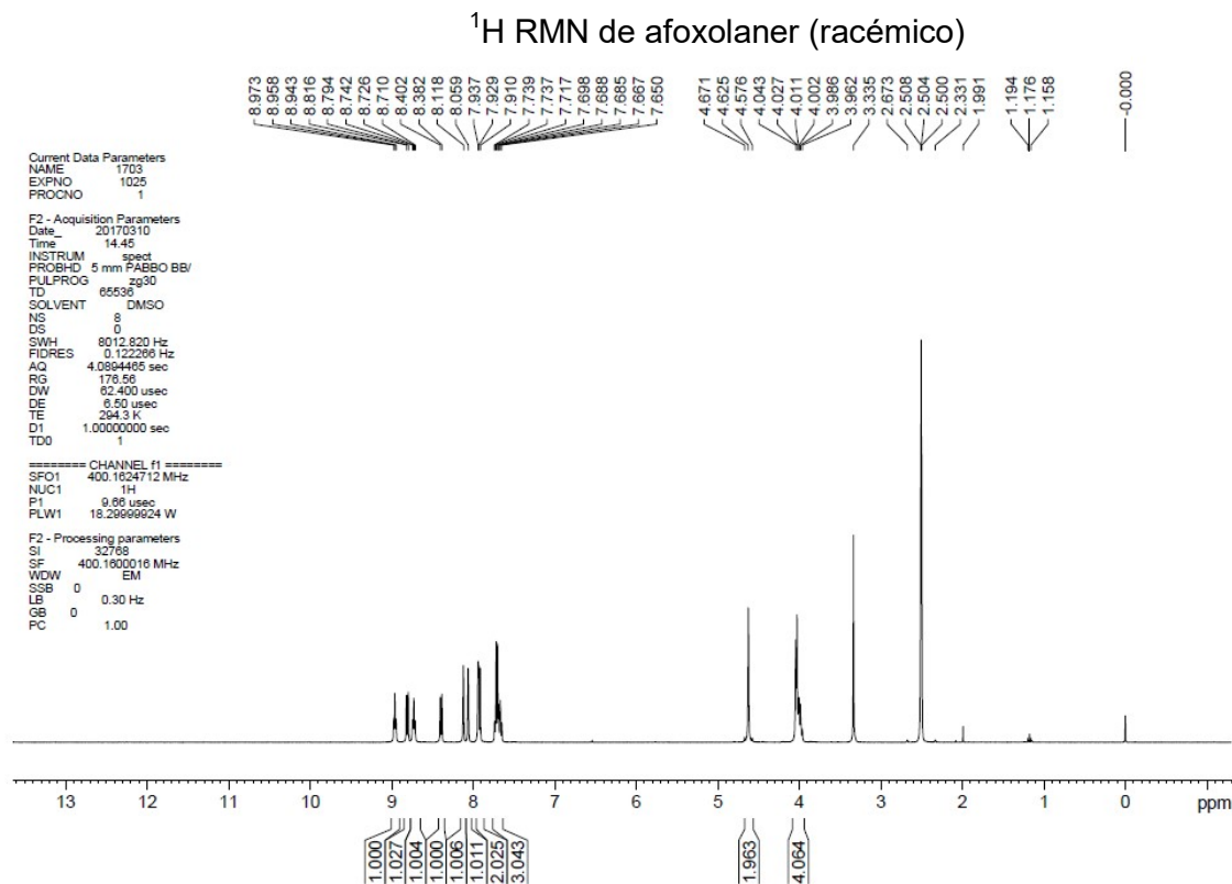
Figura 4: ^1\text{H} RMN de afoxolaner (racémico) en DMSO- \text{d}_6 .
