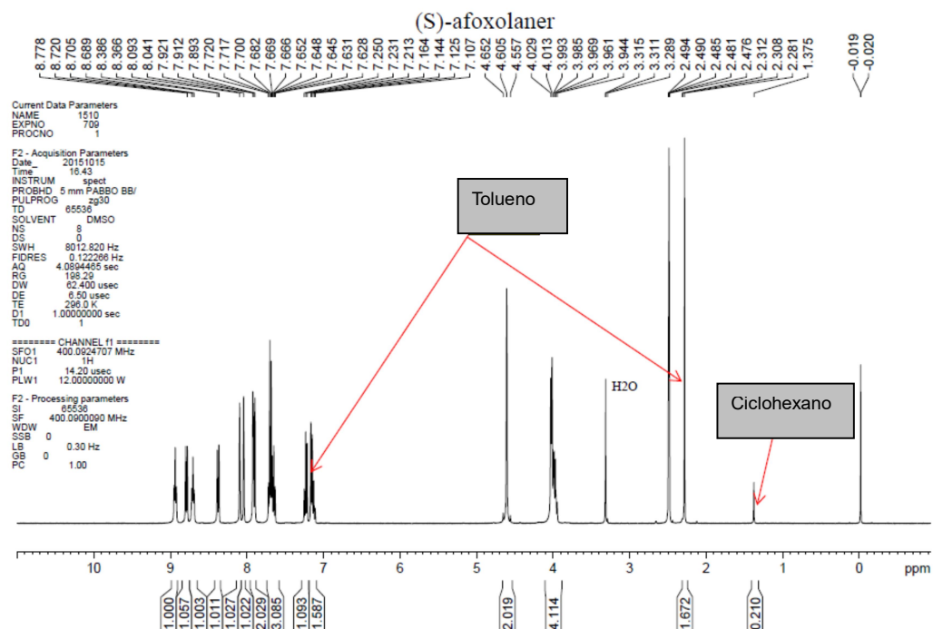
Figura 3: ^1\text{H} RMN de (S)-afoxolaner en \text{DMSO-d}_6 preparado en el Ejemplo 7
