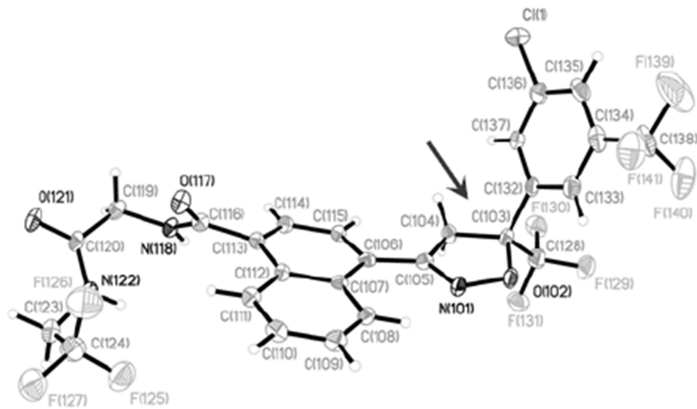
Figura 10: Estructura molecular del (S)-afoxolaner con software Cerius 2
