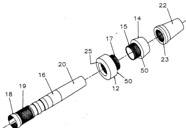
Piezas intercambiables de la boquilla del documento D3
