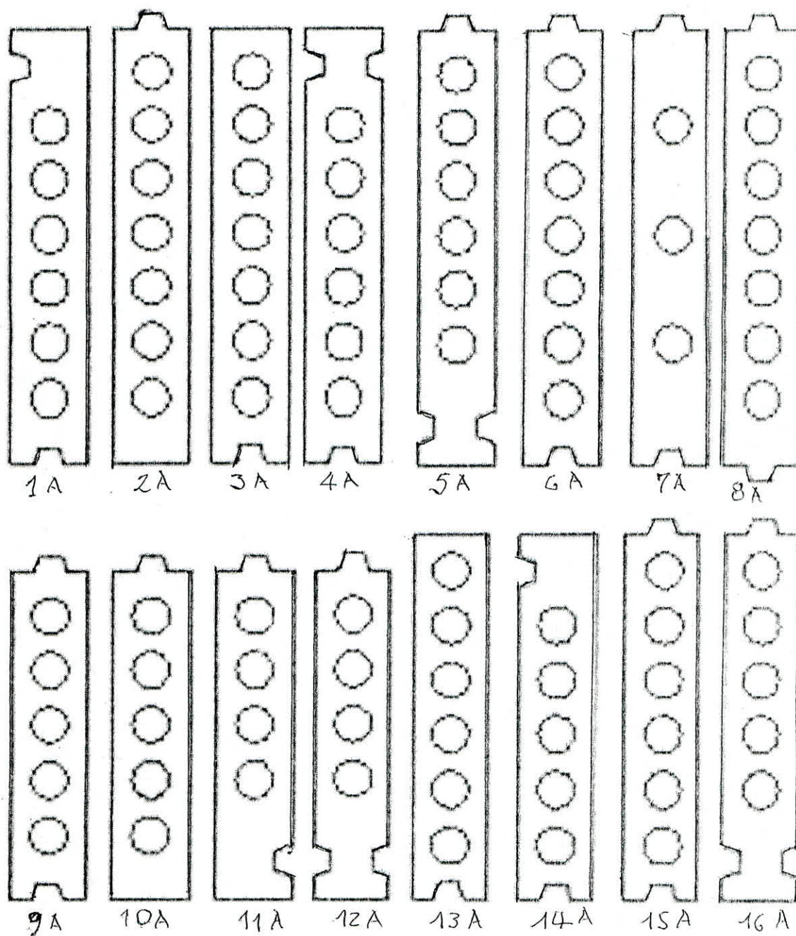
DIBUJO N° 1
