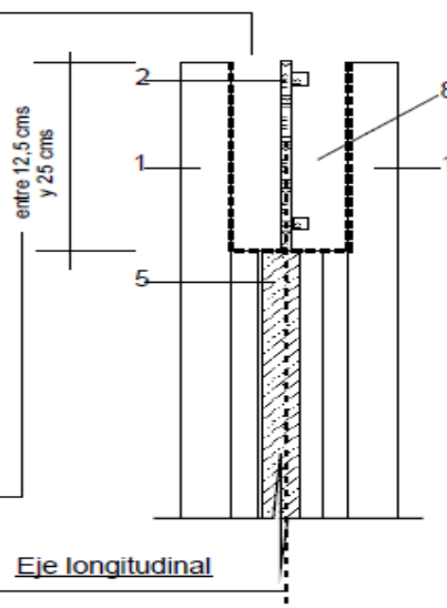
Fig. 19 Detalle ampliado corte transversal panel pared.
