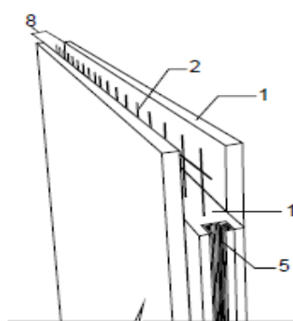
Fig. 20 Vista ampliada parte superior del panel.
