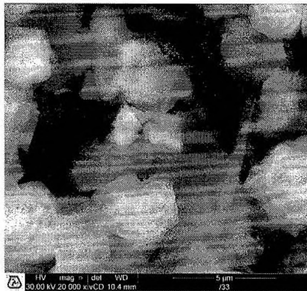
Figura 2. Imagen ESEM de la muestra del Ejemplo Comparativo 2.
