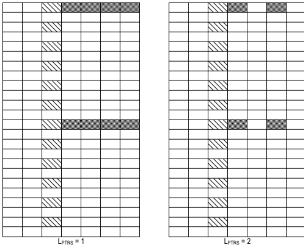
FIG. 3 Ilustración del patrón PTRS cuando K_{PTRS} = 2
