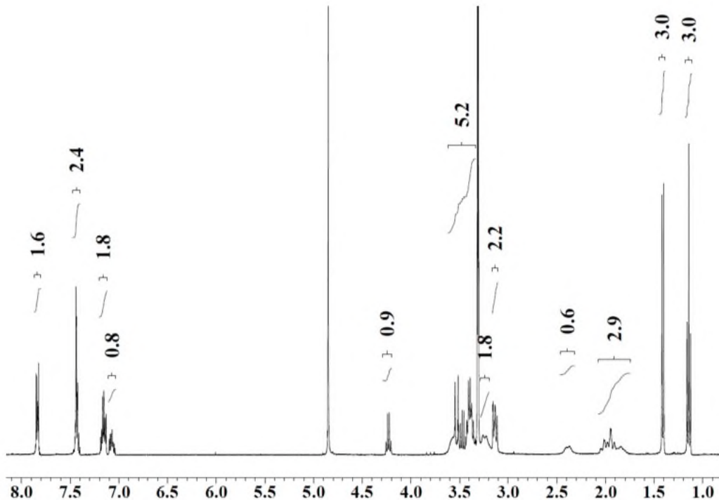
Figura 23: ^1\text{H} -RMN ( d_4 -MeOH, 400 MHz) de la sal de besilato forma P1.
