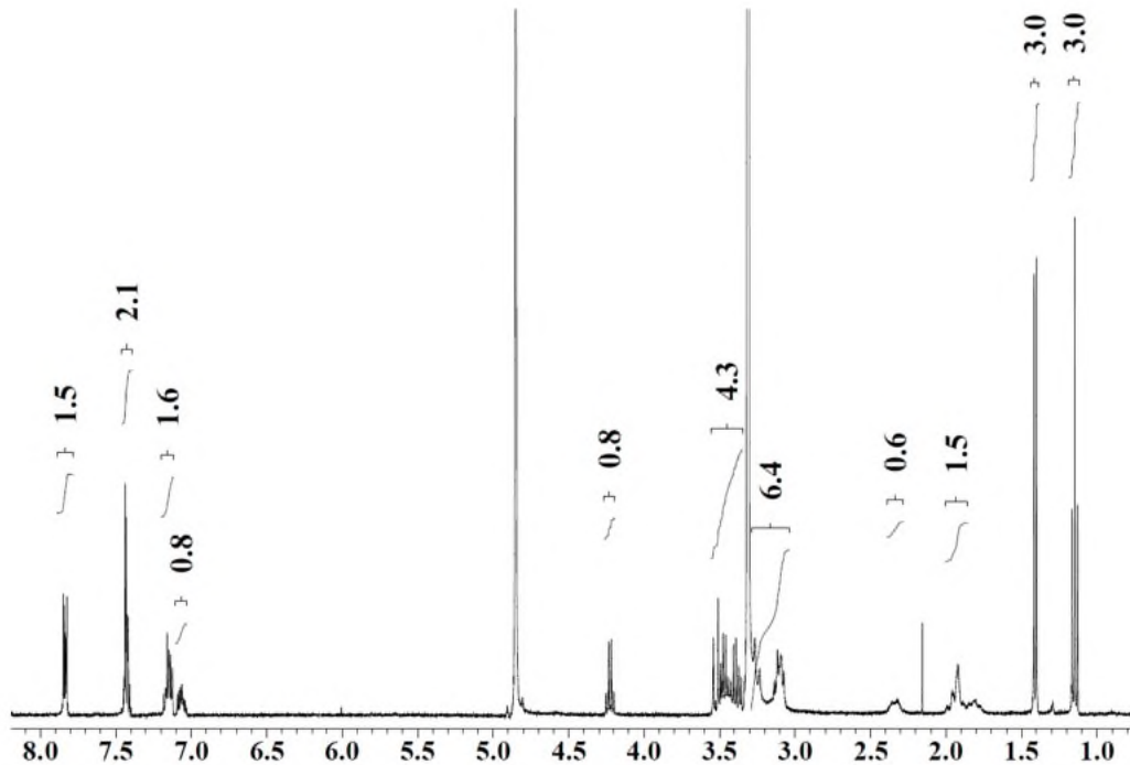
Figura 26: ^1\text{H} -RMN ( d_4 -MeOH, 400 MHz) de la sal de besilato forma P2.
