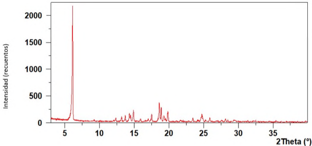
Figura 25: Patrón XRPD de la sal de besilato forma P2 obtenida con la exposición de la forma P1 a elevadas condiciones de humedad (90%).
