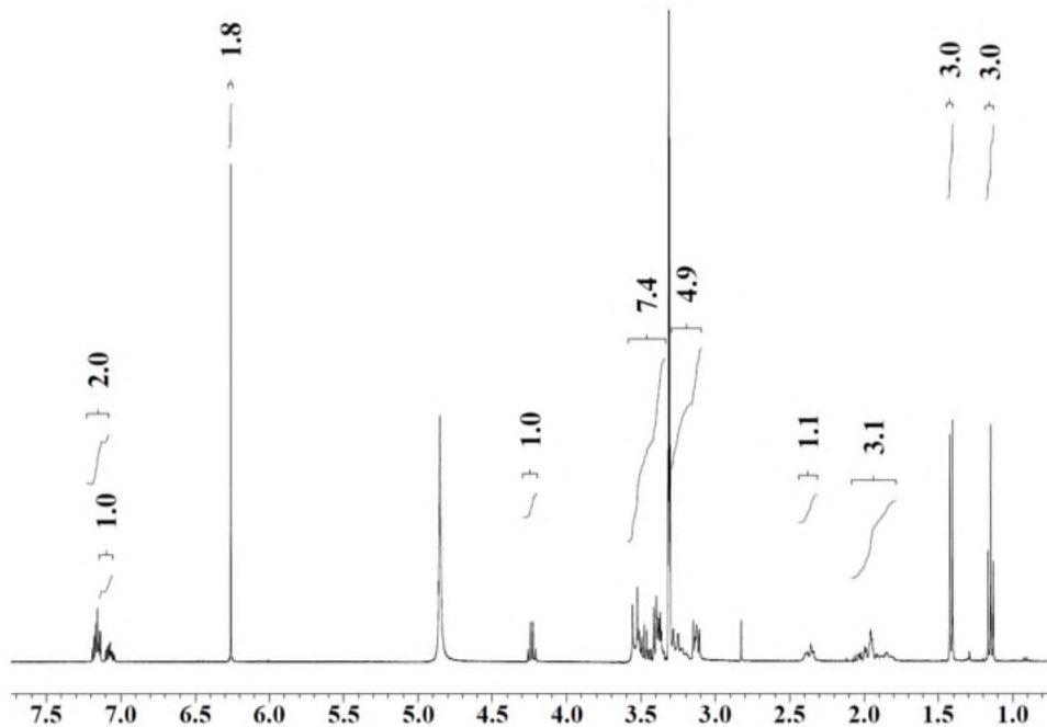
Figura 17: ^1\text{H} -RMN ( d_4 -MeOH, 400 MHz) de la sal de maleato forma P2.
