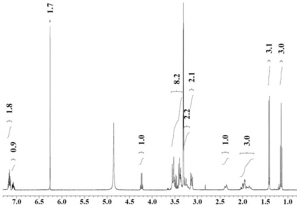
Figura 20: ^1\text{H} -RMN ( d_4 -MeOH, 400 MHz) de la sal de maleato forma P3.
