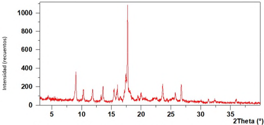
Figura 19: Patrón XRPD de la sal de maleato forma P3 obtenida por precipitación en IPA.
