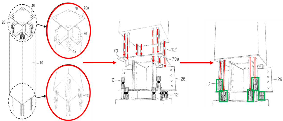
Figura 2-Modalidad de D1 donde se unen las barras de las columnas por medio de conectores
