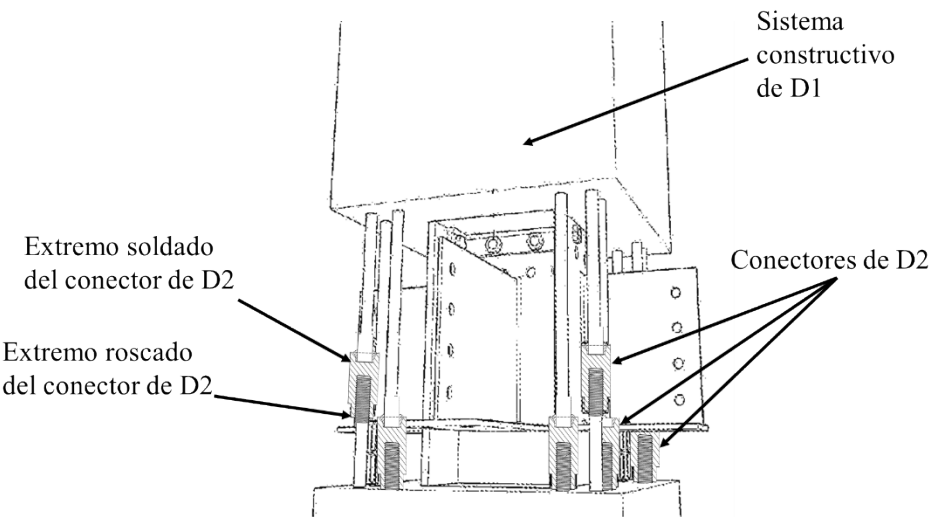
Figura 4-Producto de la combinación de D1 y D2
