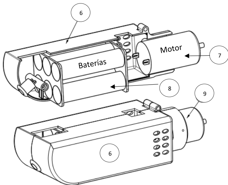
Figura 2. Carcasa de batería y motor
