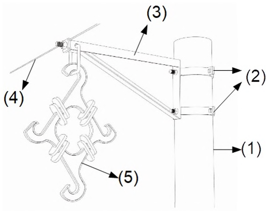
Figura 1. Vista general del dispositivo soporte tangencial integral, instalado en el poste con el espaciador polimérico.
