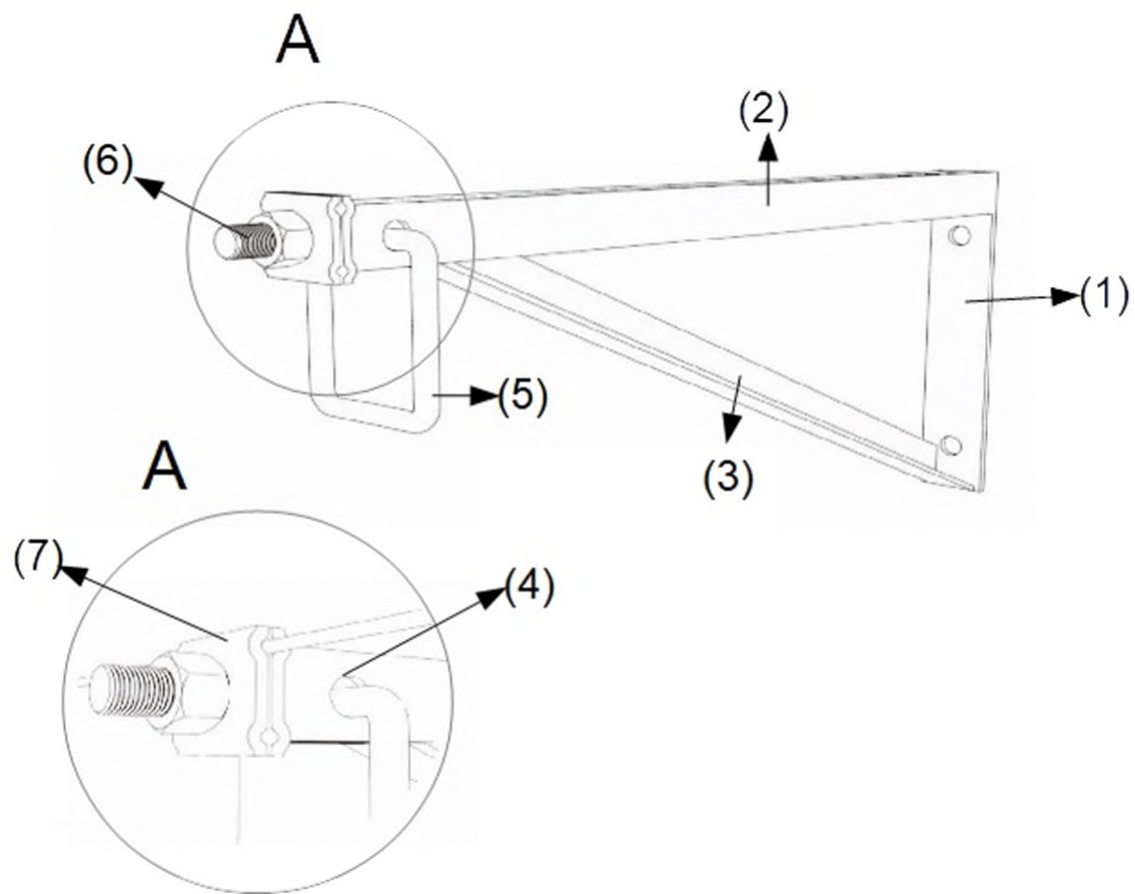
Figura 2. Vista lateral del Dispositivo de soporte con estribo integrado, con sus respectivos componentes.
