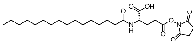
Moiety B-OSu
