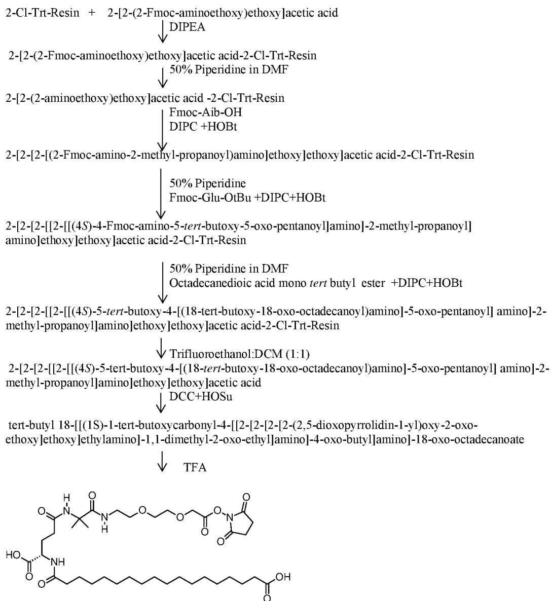
Moiety D-OSu
