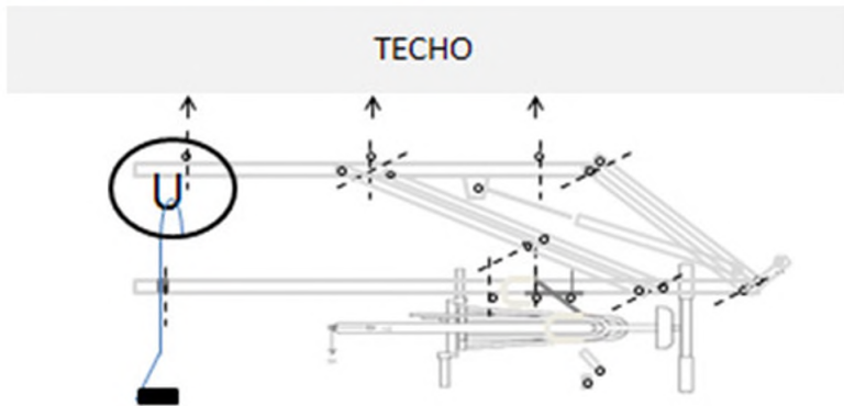
Grafica 12 – Sistema Fijación tubo superior:
