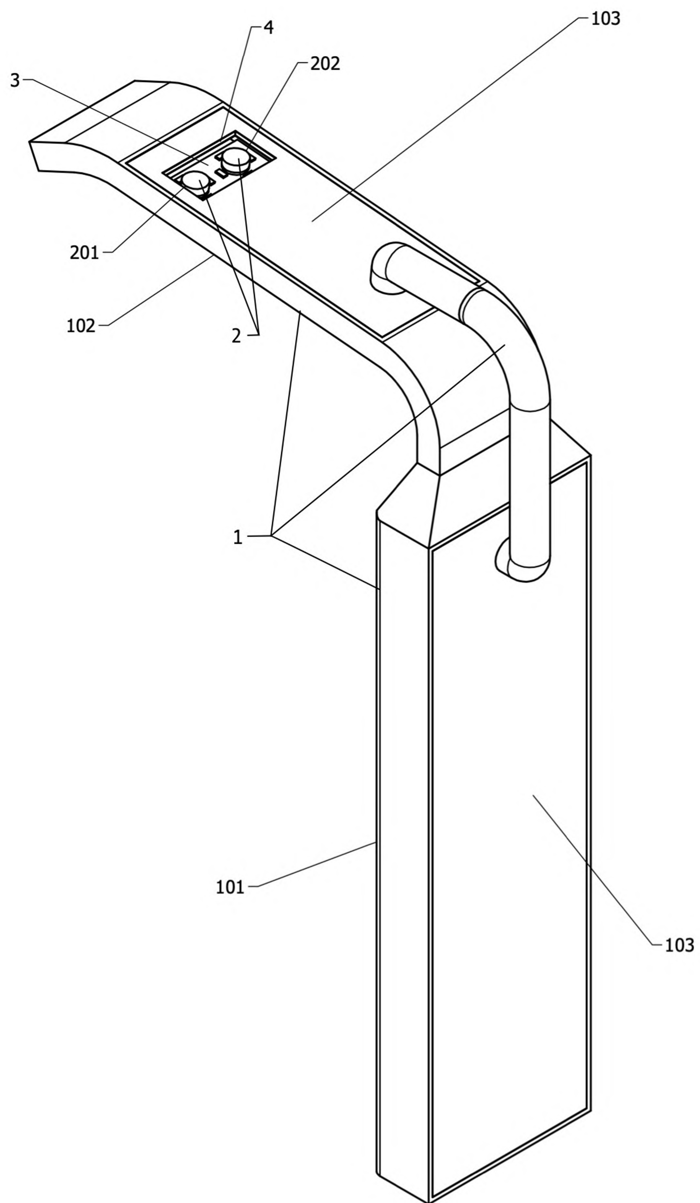
Figura 1. Dispositivo retractor ensamblado, vista isométrica.
