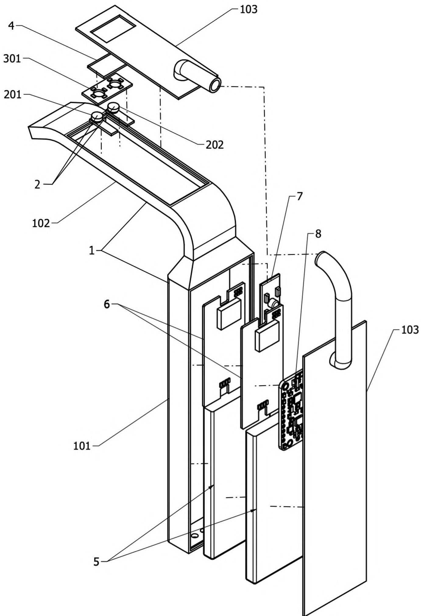
Figura 2. Componentes principales del dispositivo, vista isométrica.
