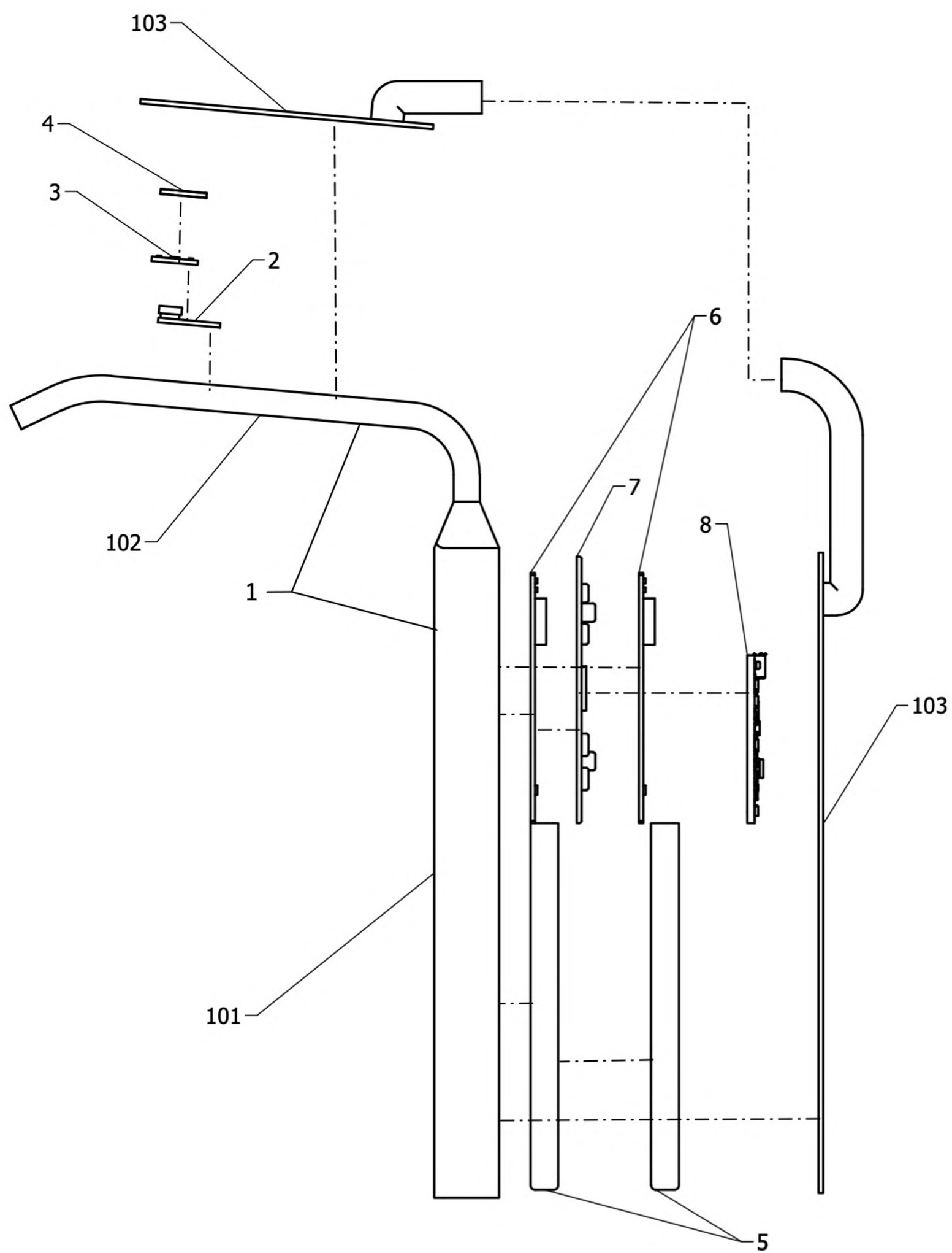
Figura 3. Componentes principales del dispositivo, vista Lateral.
