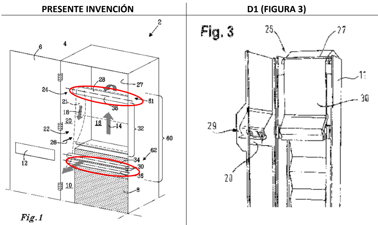
Figura 1: comparación gráfica del dispensador (2) de la presente invención (Figura 1 del Capítulo Descriptivo) y el dispensador de D1 (Figura 3 de D1).
