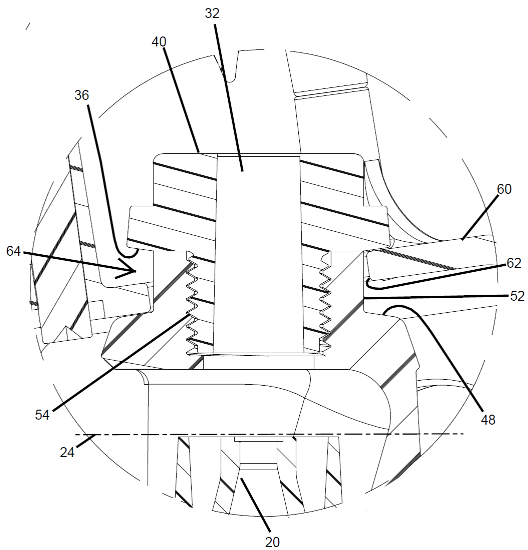
Detalle 7A
