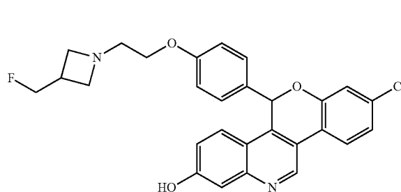
5-(4-{2-[3-(fluoromethyl)azetidin-1-yl]ethoxy}phenyl)-7-(trifluoromethyl)-5H-[1]benzopyrano[4,3-c]quinolin-2-ol
