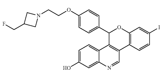
8-fluoro-5-(4-{2-[3-(fluoromethyl)azetidin-1-yl]ethoxy}phenyl)-5H-[1]benzopyrano[4,3-c]quinolin-2-ol
