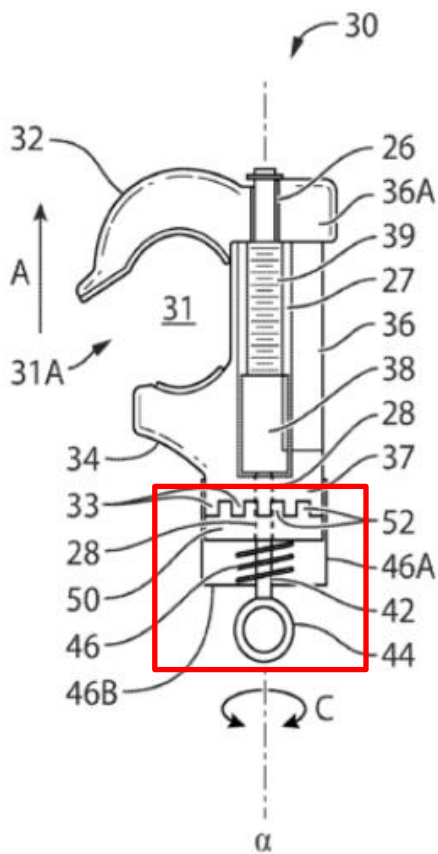
Figura 1. Acoples y bloqueo en presente invención.
