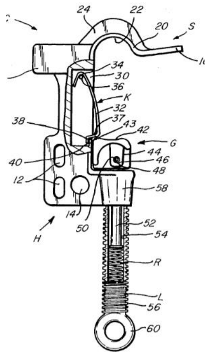
Figura 2. Abrazadera en D1.
