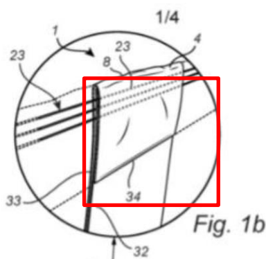
Figura 1. Doblado o elemento elástico emparedado de la presente invención
