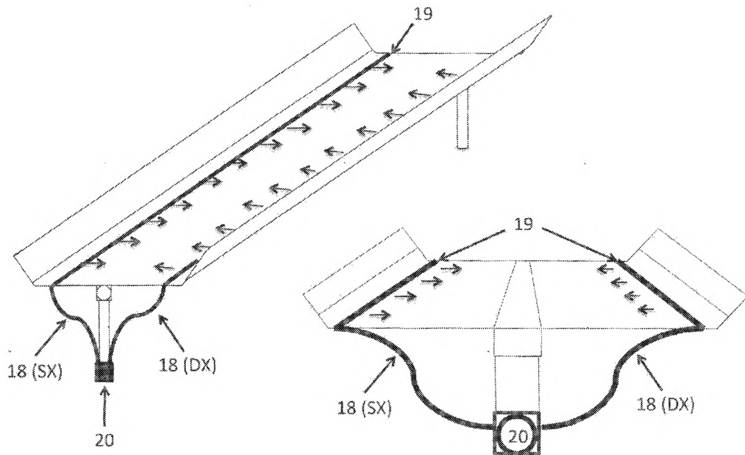
FIG. M The Double Circuit Water System n.17
