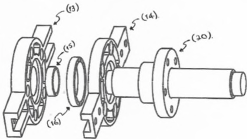
Figura 6. Estructura de apoyo a los ejes
