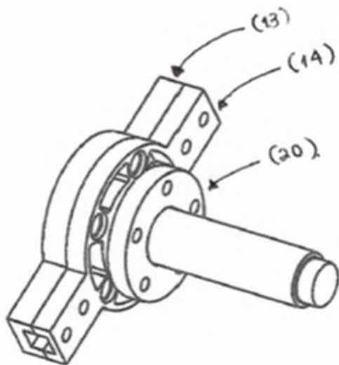
Figura 7. Estructura de apoyo a los ejes ensamblada
