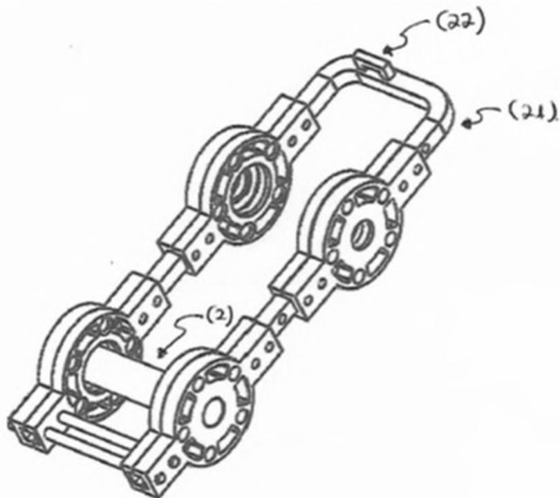
Figura 8. Módulo estructural
