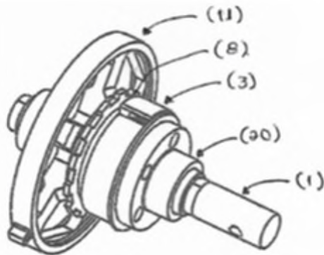
Figura 10. Alineación de componentes sobre uno de los ejes
