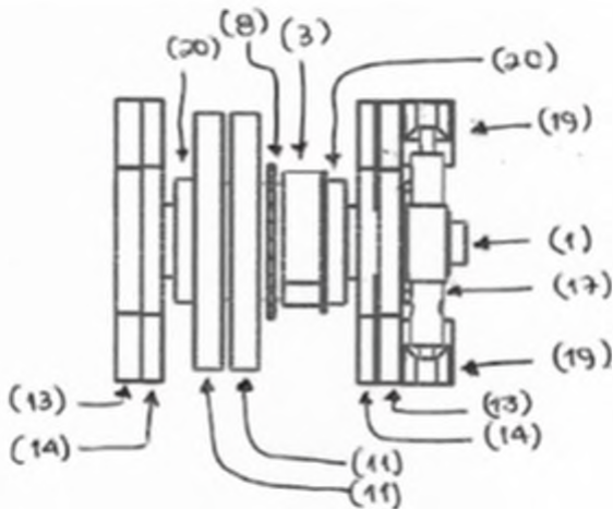
Figura 12. Alternativa con doble polea de usuario
