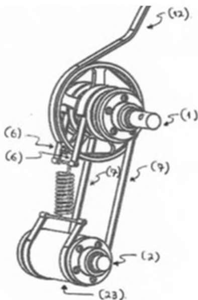
Figura 13B - Alternativa con ejes colineales - Vista inclinada
