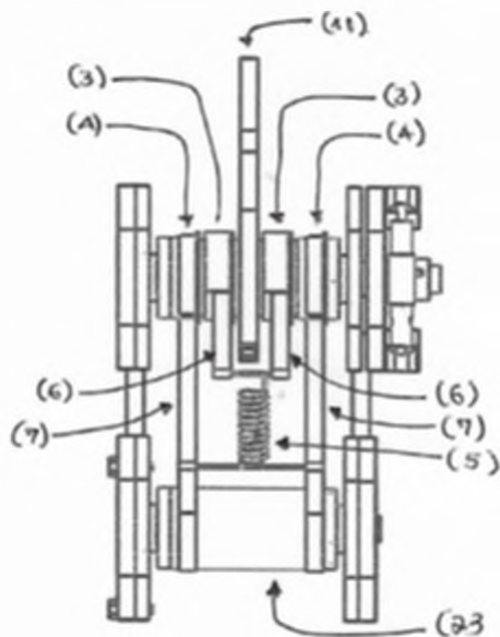
Figura 13A - Alternativa con ejes colineales - Vista alineación
