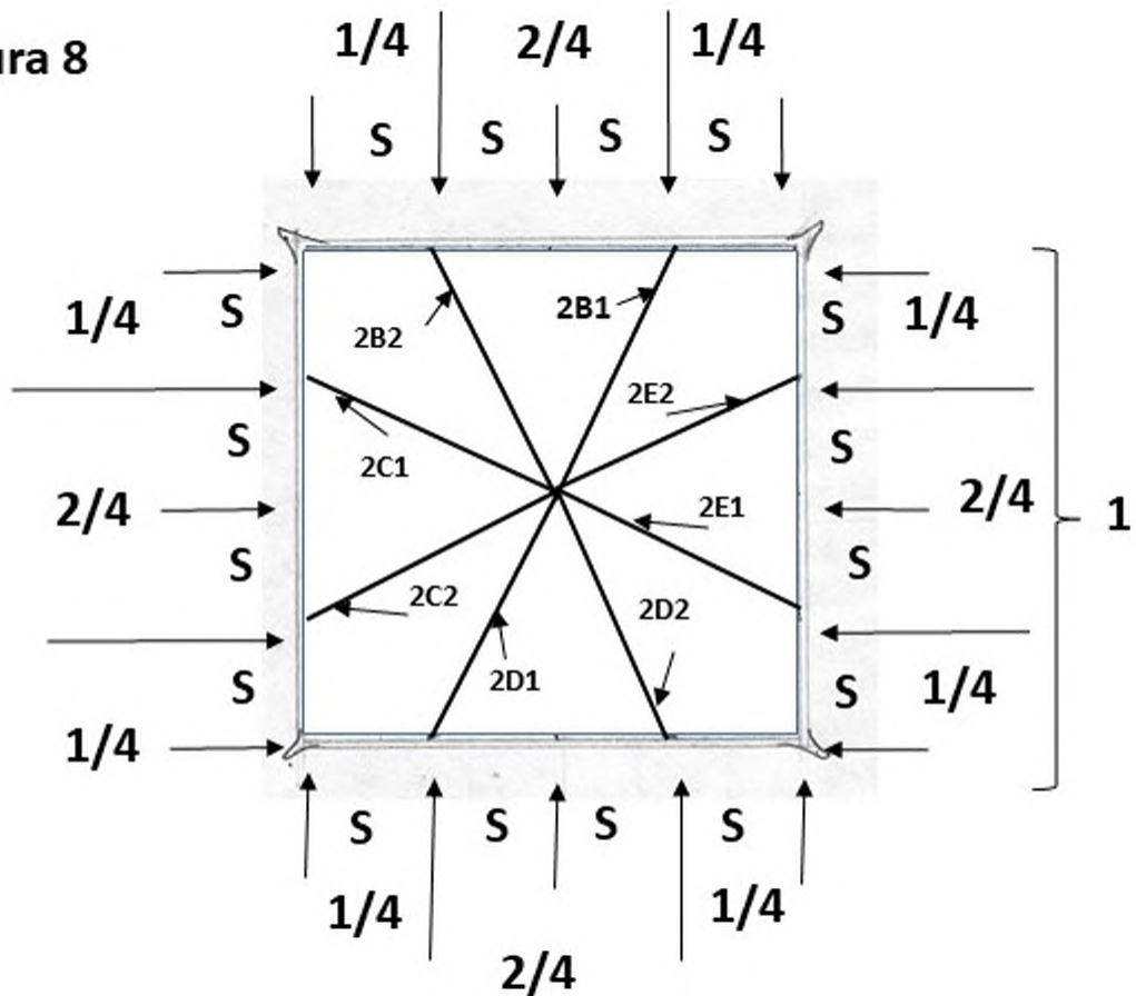
Figura 8. Se muestra en vista frontal, la ubicación de los cuatro módulos de las mallas en "V" (2B), (2C), (2D) y (2E) en el interior del saco contenedor (1) y su relación con las secciones (S), (2/4 y 1/4)
