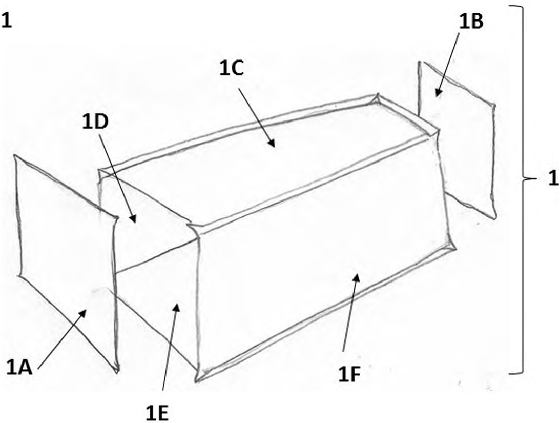
Figura 11. Se muestran en una perspectiva y en despiece; las telas o caras frontal y posterior (1A) y (1B) y las telas o caras laterales (1C), (1D), (1E) y (1F) del saco contenedor (1).
