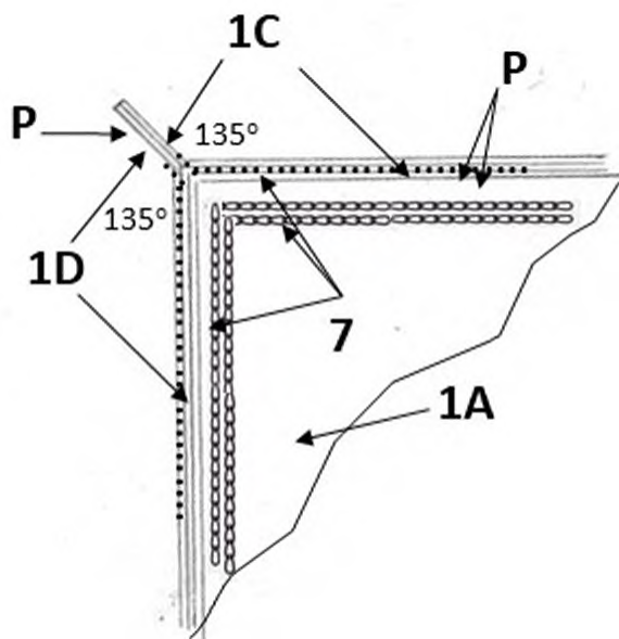
Figura 12. Se muestra en un corte de sección en vista superior, la proyección exterior (P) a dos ángulos de 135°, en la ubicación de las caras o telas laterales (1C), (1D) y (1A) con sus costuras (7).
