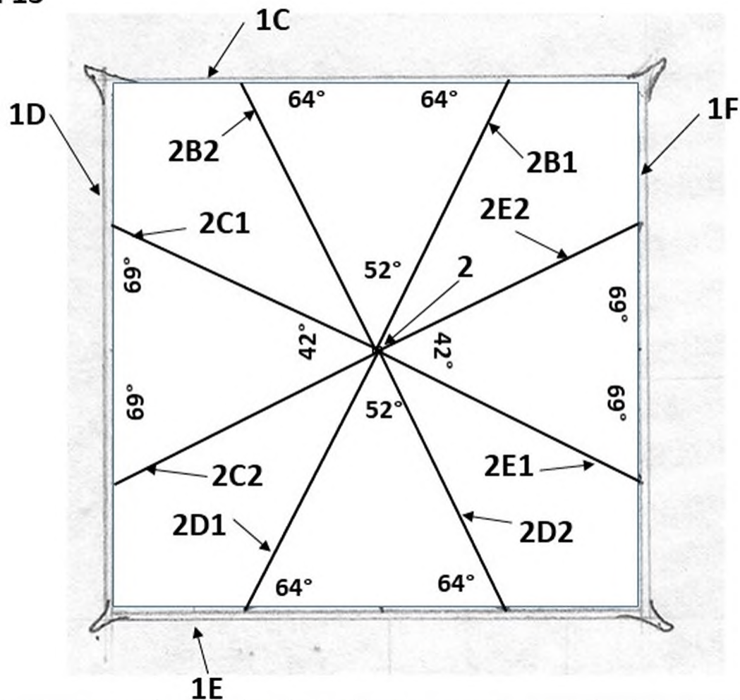
Figura 13. Se aprecian en vista frontal las caras o telas (1C), (1D), (1E) y (1F) y en el cuerpo de malla de tensión interna (2), los ángulos alternos-internos de 64° formados por las secantes de las mallas en "V" (2B1 y 2B2) y de (2D1 y 2D2) con sus ángulos alternos internos de 52°, así como los ángulos alternos-internos de 69° formados en los módulos de las mallas en "V" (2C1 y 2C2) y (2E1 y 2E2) con sus ángulos alternos internos de 42°.
