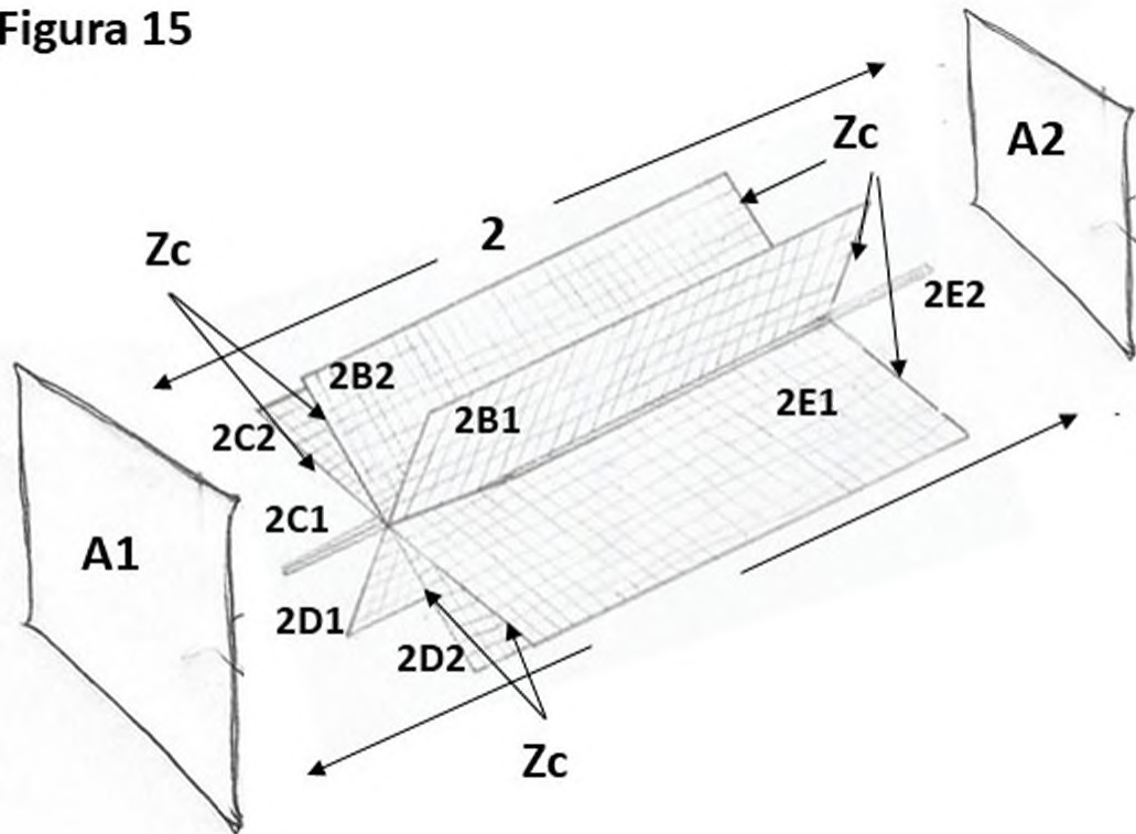
Figura 15. Muestra en perspectiva la unión de las caras o telas (1A) y (1B) del cuerpo de malla de tensión interna (2) con sus secantes de las mallas en "V" (2B1 y 2B2), (2C1 y 2C2), (2D1 y 2D2) y (2E1 y 2E2). Aparecen las Zonas de canto (Zc).
